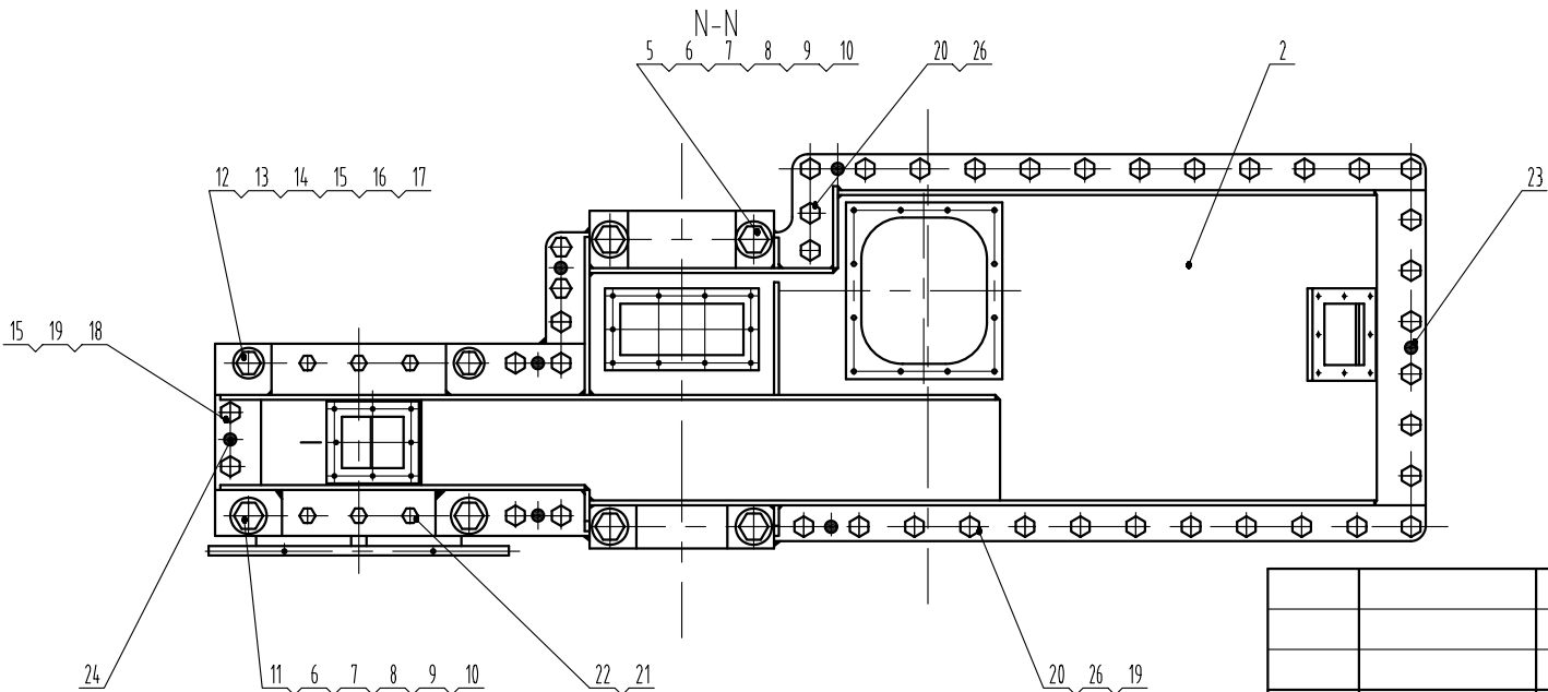
Болт и фиксирующий штифт на крышке шестеренчатой коробки как показано на схеме 齿轮箱上螺栓、定位销示意图
