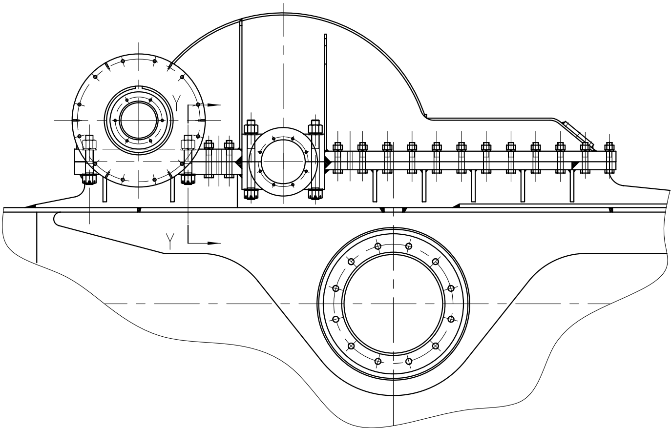
Болт и фиксирующий штифт на крышке шестеренчатой коробки как показано на схеме 齿轮箱上螺栓、定位销示意图
